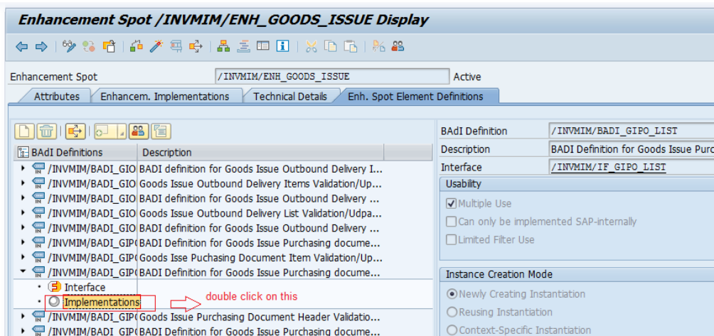
Figure 10-6 BADI: /INVMIM/BADI_GIPO_LIST
